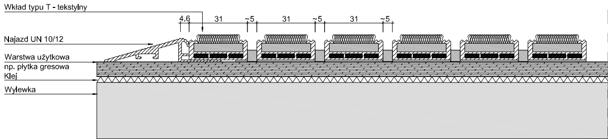
UNIMAT 12 T_M + UN 10/12
