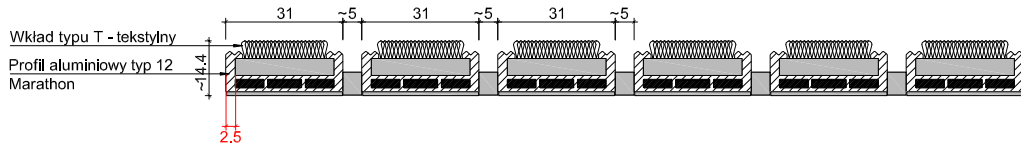
UNIMAT 12 T_M + UN 10/12
